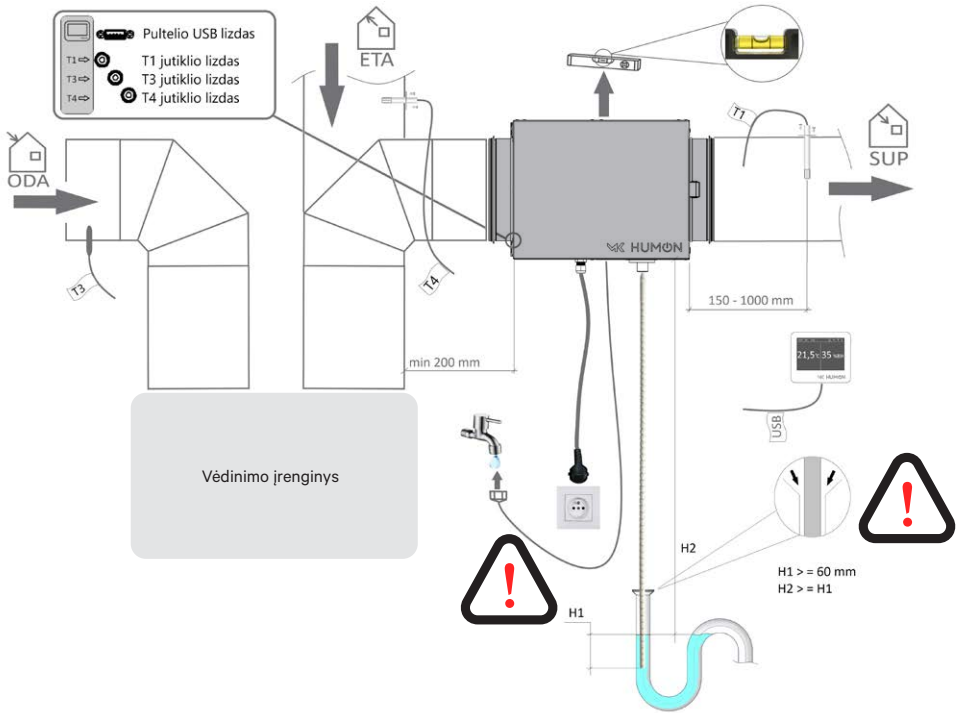
4 pav. HUMON drėkintuvo montavimo schema
