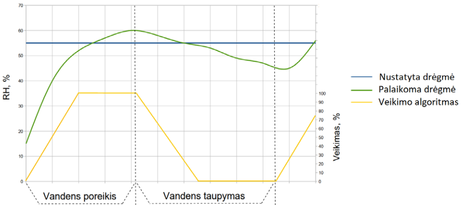
8 pav. Darbo principo diagrama
