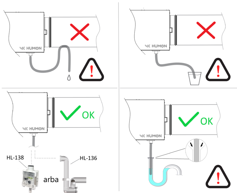
5 pav. Drenažo įrengimo schemas
