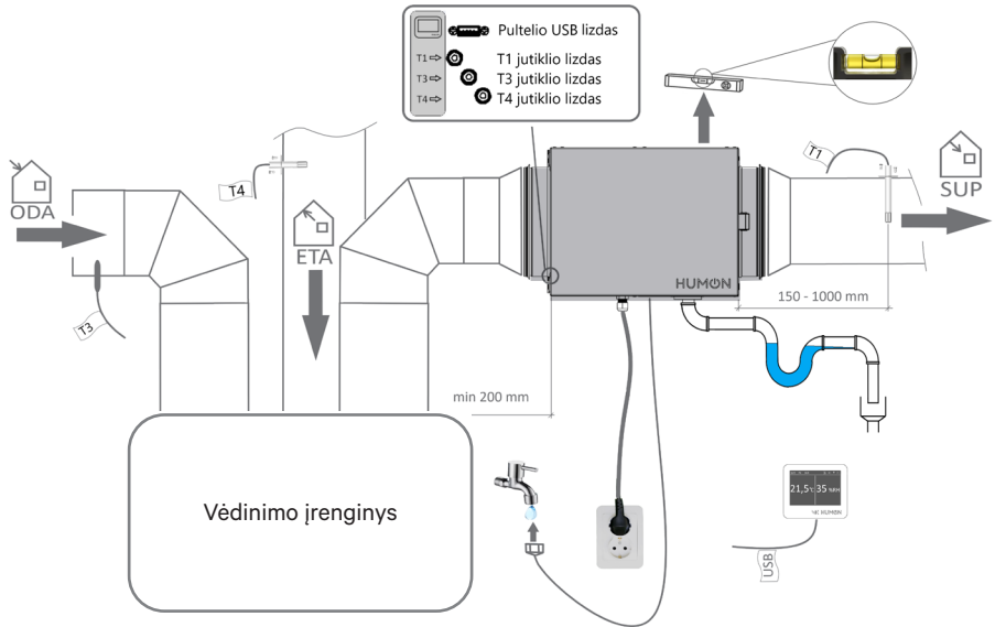
Drėkintuvų H200, H250, H315 montavimo schema
